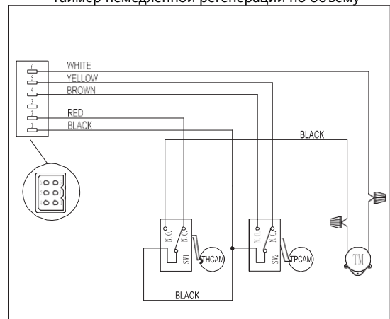
Таймер немедленной регенерации по объему
