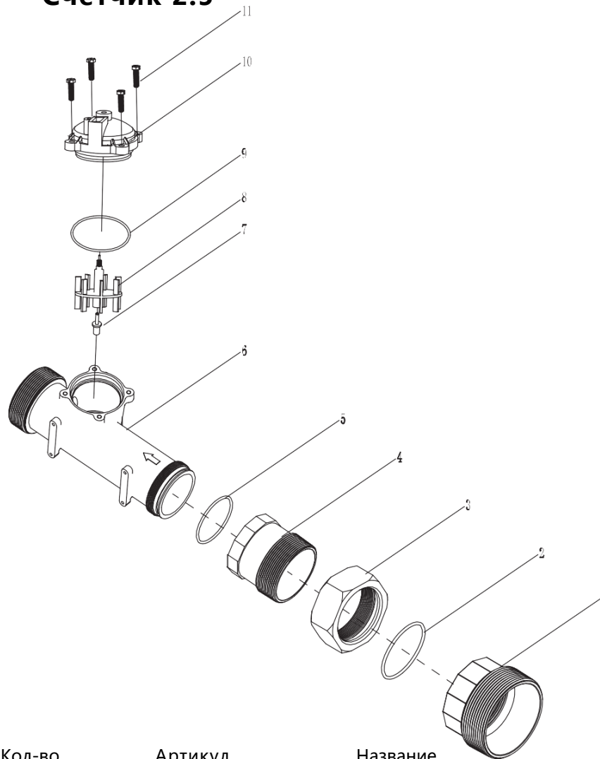
Счетчик 2.5"
